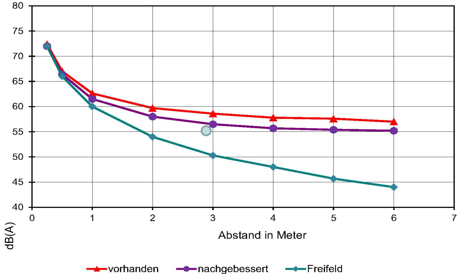
Schallpegelverteilung
